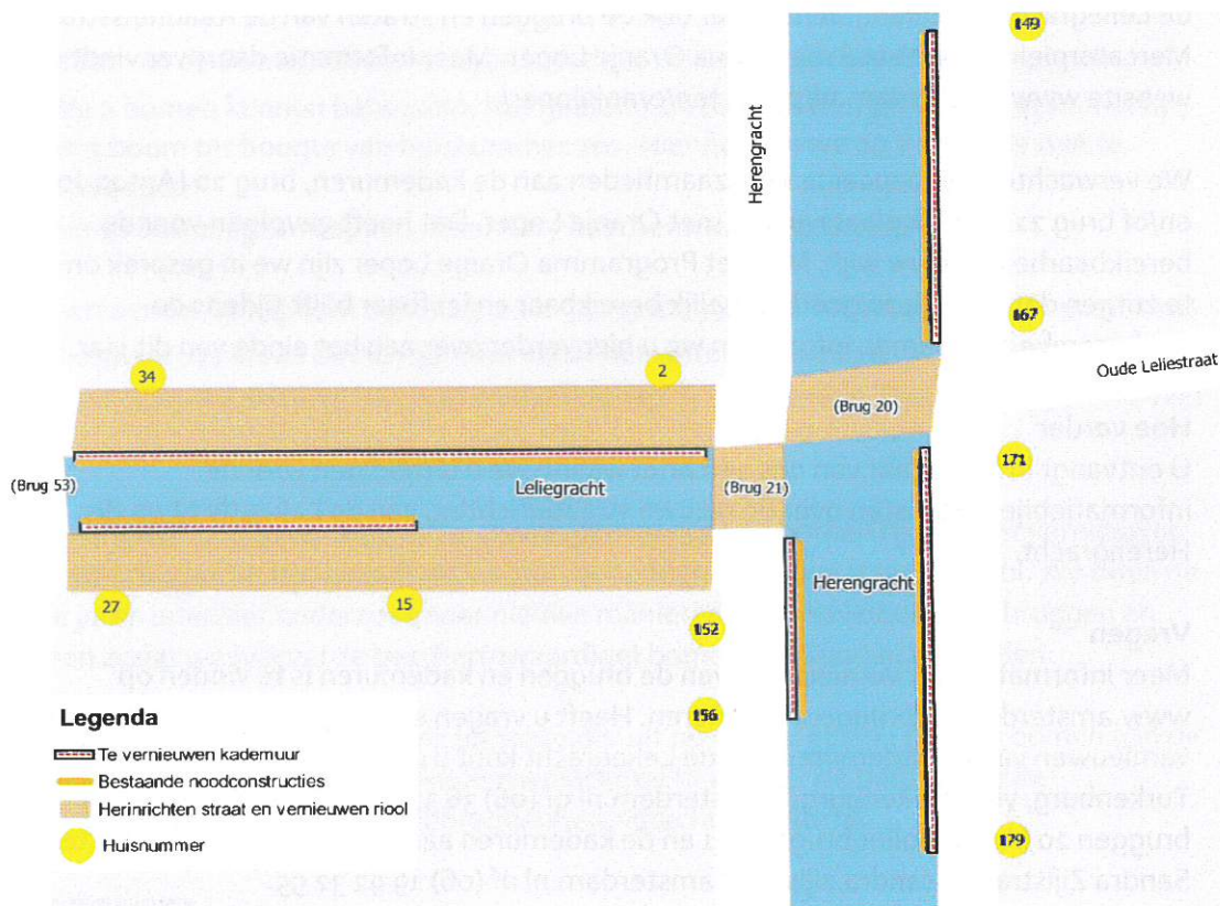
Werkgebied kademuuren Leliegracht/Herengracht en bruggen 20 en 21
